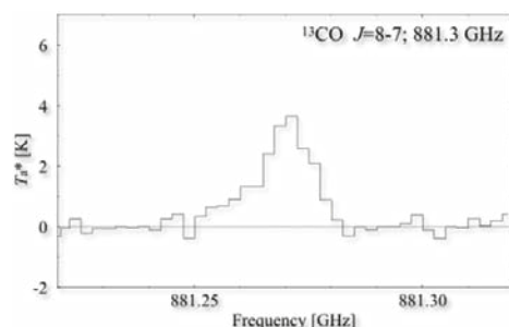
図 3 製作した受信機でオリオン座分子雲で検出した一酸化炭素分子のスペクトル
