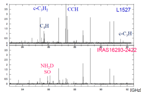
図 2 L1527 と IRAS16293-2422 の比較。後者は Caux et al. (2011) を引用。
